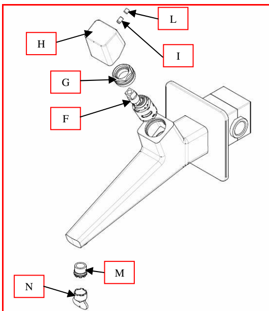
FIGURA 5 - MONTAGGIO GRUPPO RUBINETTO
