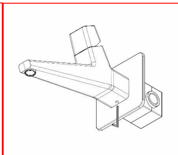
FIGURA 4 - FISSAGGIO GRUPPO RUBINETTO.
